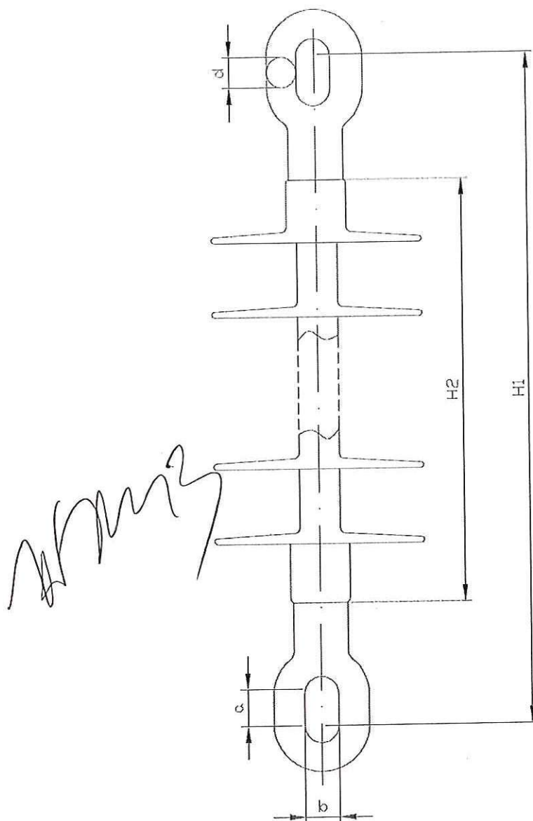
Фигура 2 – Композитен висящ изолатор, тип „ухо-ухо“
