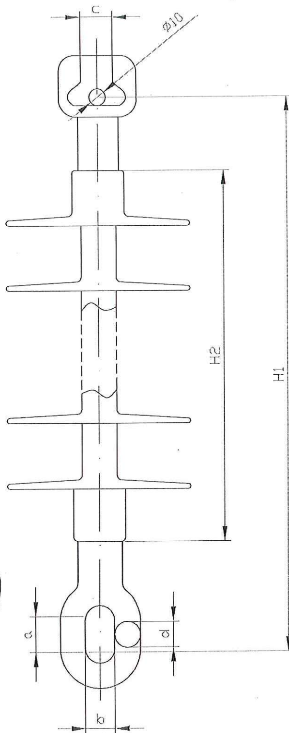
Фигура 1 – Композитен висящ изолатор, тип “ухо-кратунка”
